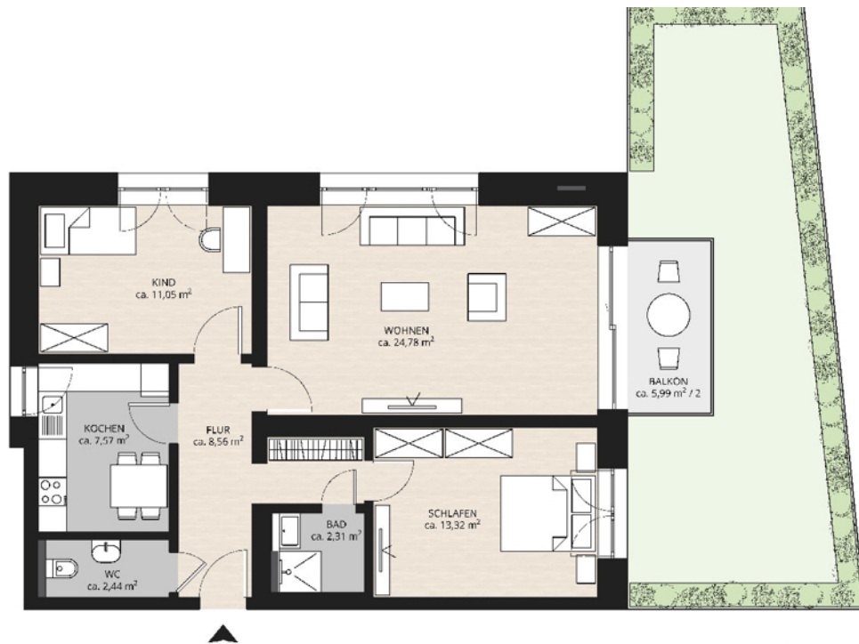
Grundriss Wohnung 2
