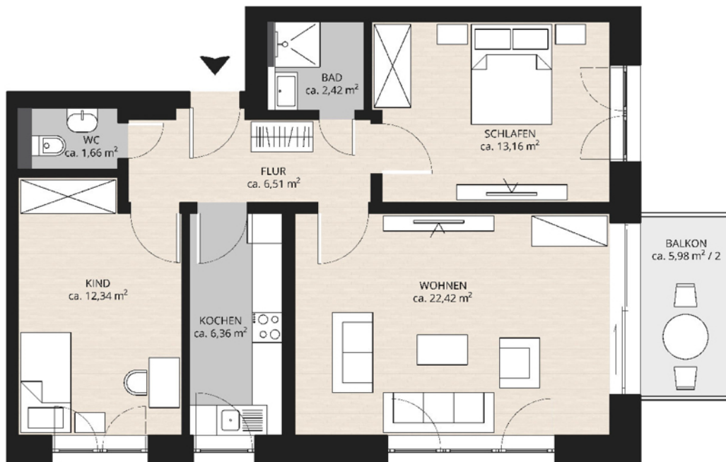
Obergeschoss - Wohnung 6
