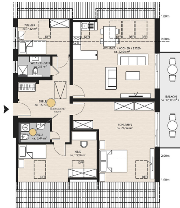
Dachgeschoss - Wohnung 8
